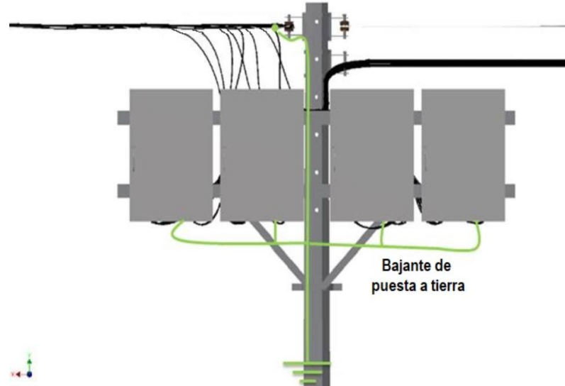
Figura 5. Sistema de puesta a tierra para la medida semi-concentrada.
