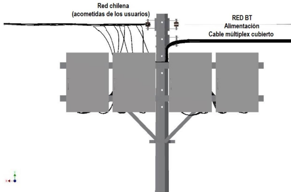
Figura 2. Montaje de medida semi-concentrada
