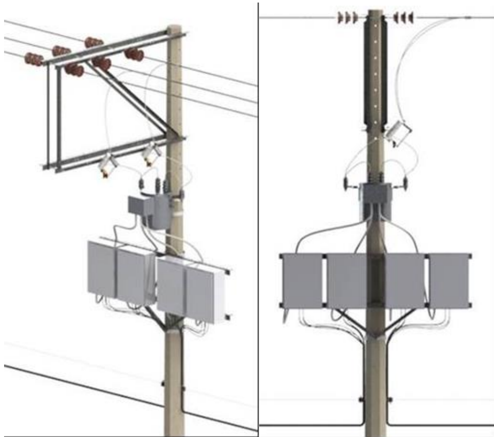
Figura 1. Montaje de medida concentrada con transformador de frente muerto.
