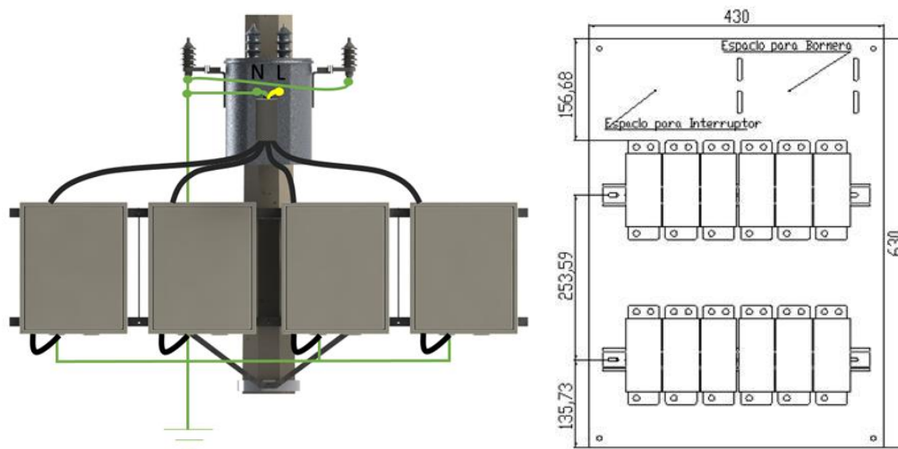
Figura 4. Sistema de puesta a tierra para la medida concentrada.
