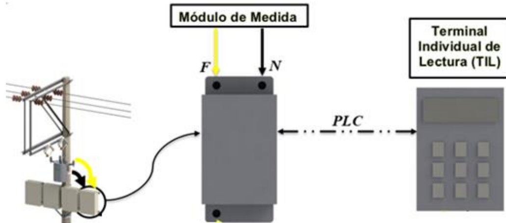
Figura 9. Esquema de conexión del módulo de medida y el terminal individual de lectura con comunicación PLC
